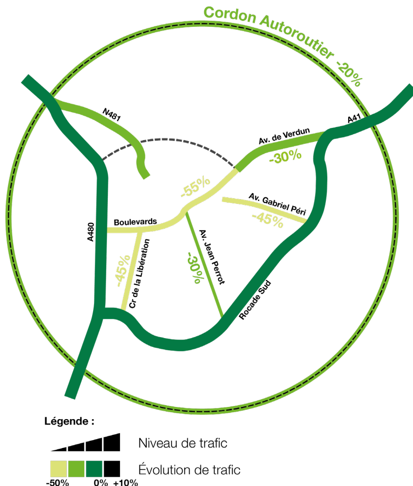
Figure 2 Synthèse de la baisse de trafic sur l'aire urbaine grenobloise de 1996 à 2018
